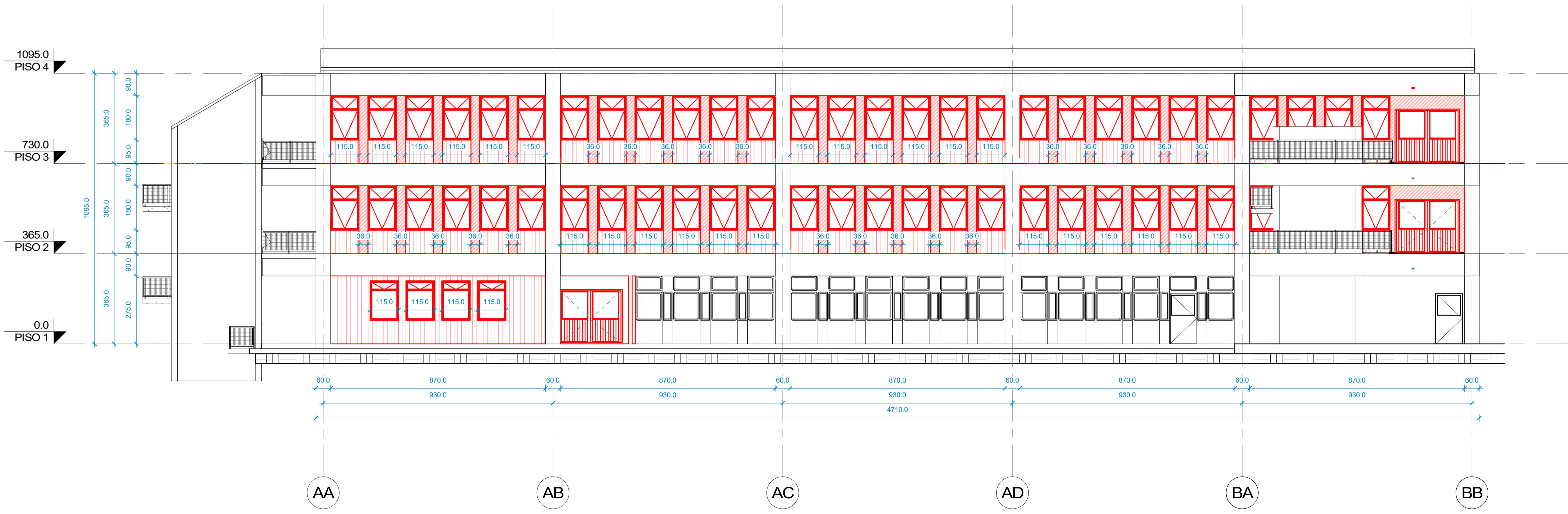
2 ELEV P - PA- PROYECTADO 1 : 100
