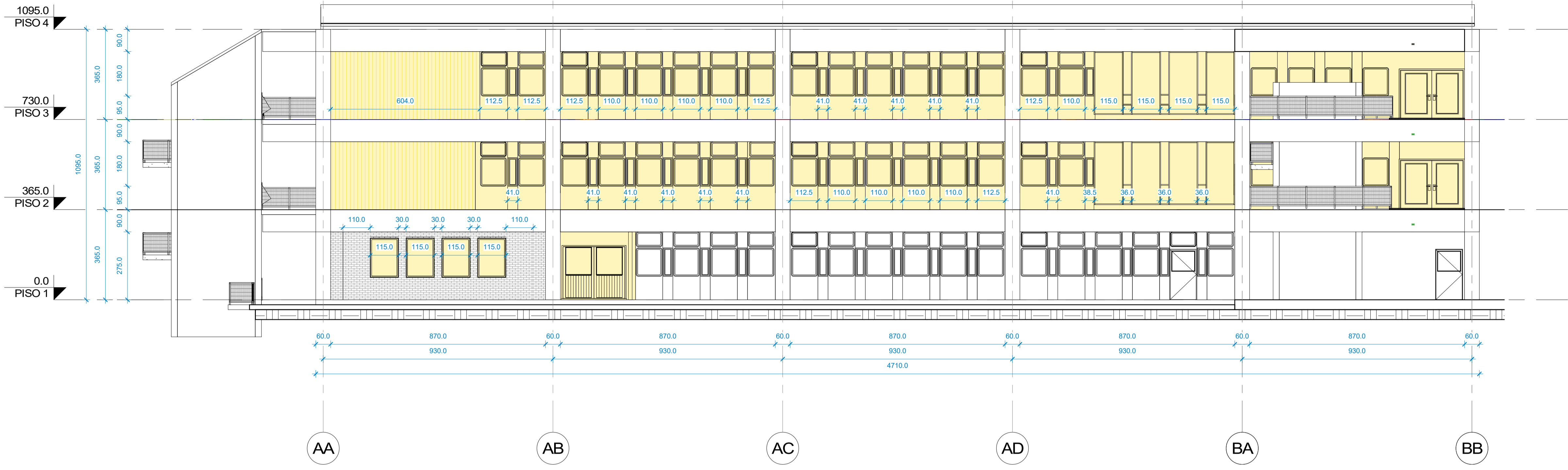
1 ELEV P - PA- DEMOLICIÓN 1 : 100
