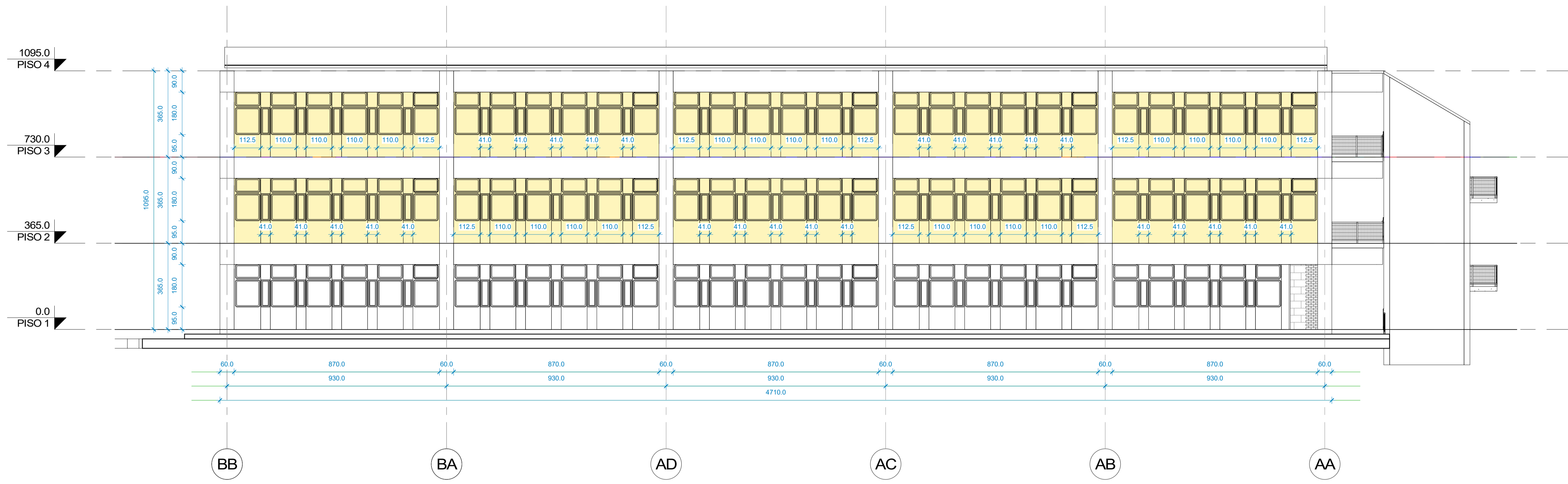
1 ELEV O - PA - DEMOLICIÓN 1 : 100
