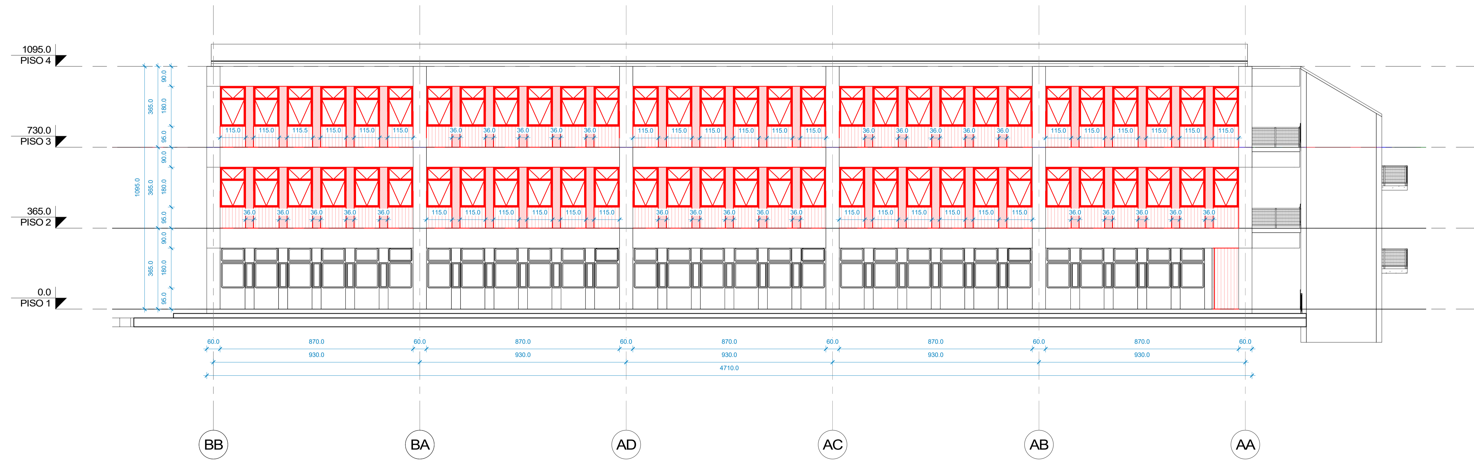
2 ELEV O - PA - PROYECTADO 1 : 100
