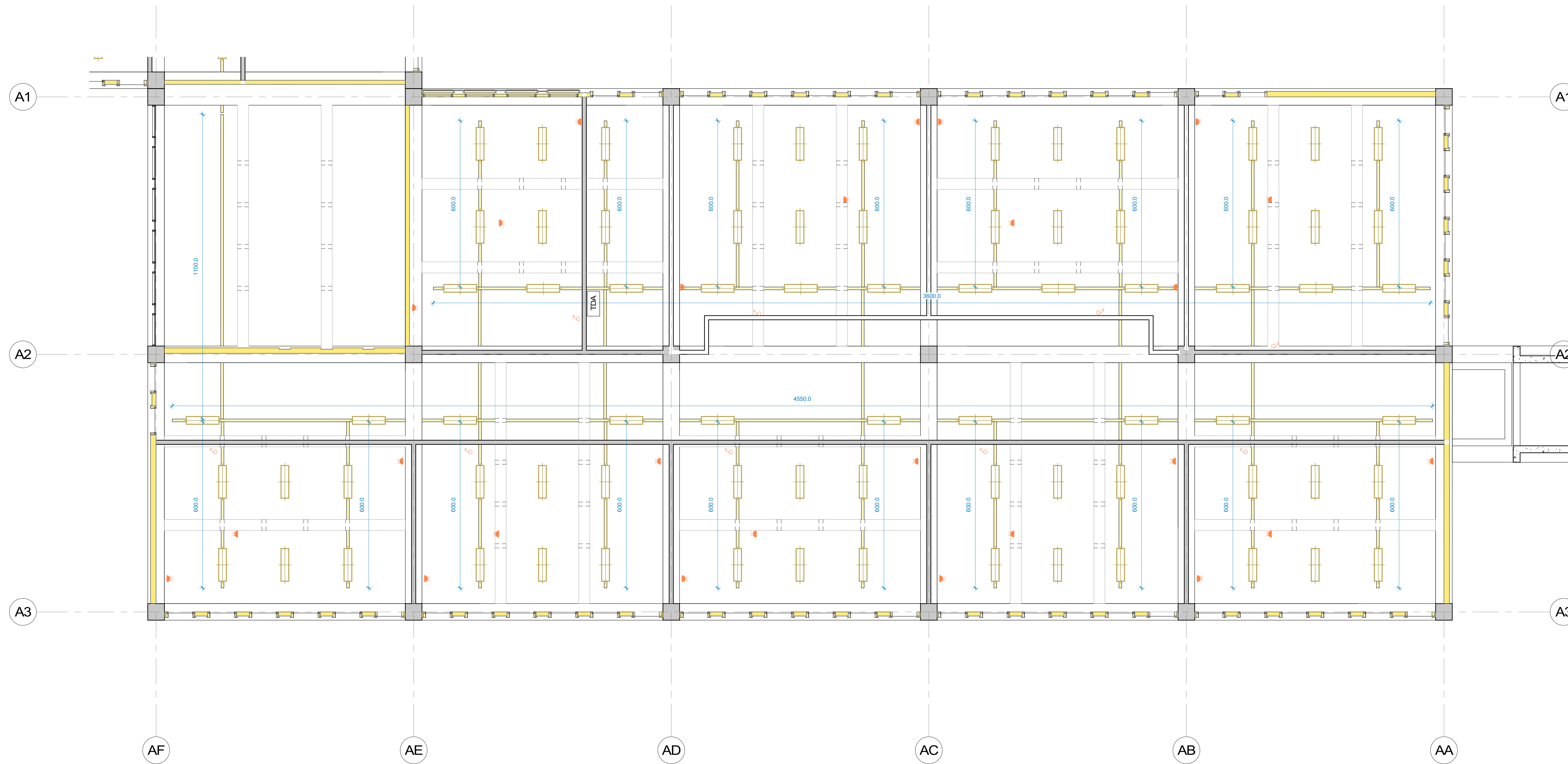
1 CIELO 3 - PA - DEMOLICIÓN 1 : 75
