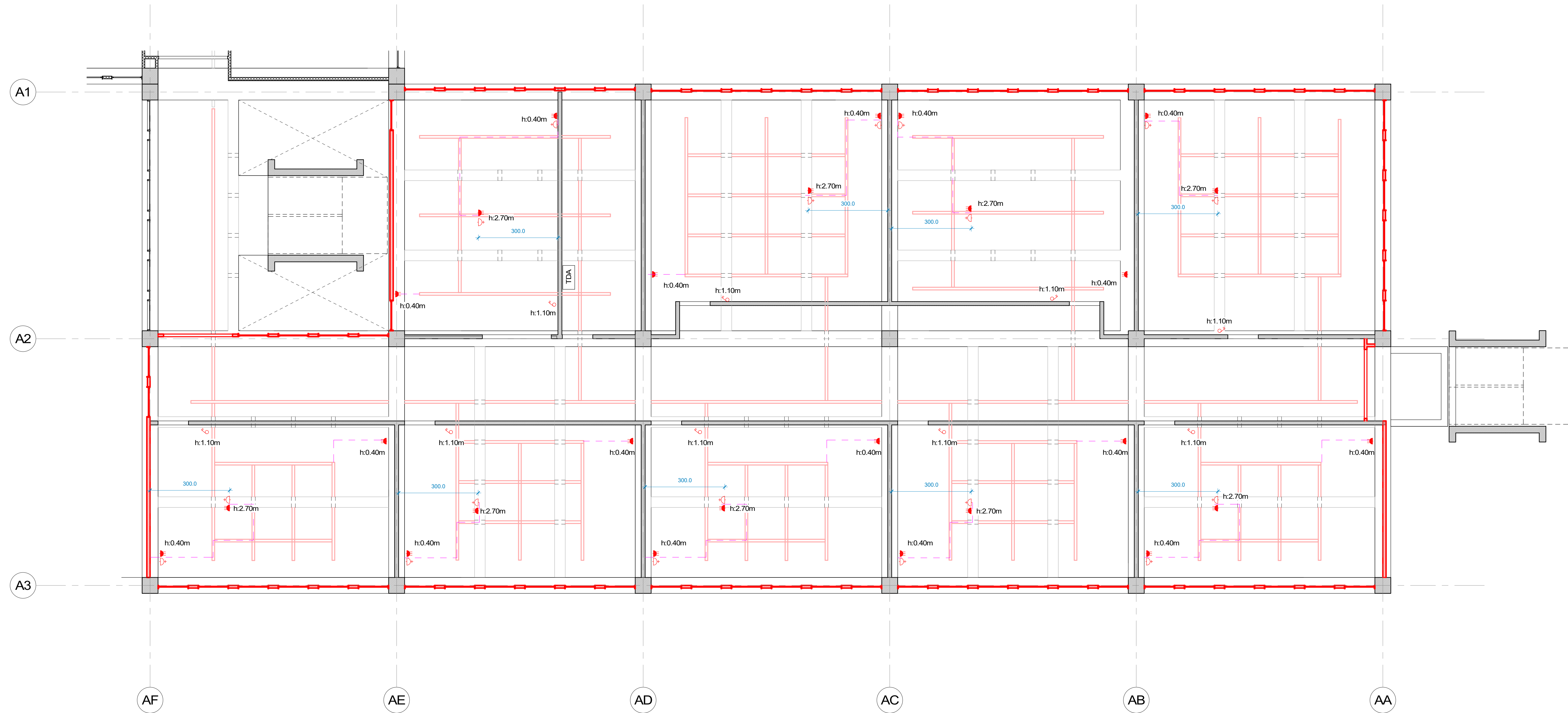
1 CIELO 2 - PA - PROPUESTA ENCHUFES 1 : 75
